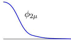
Fig. 4. Half a soliton.
